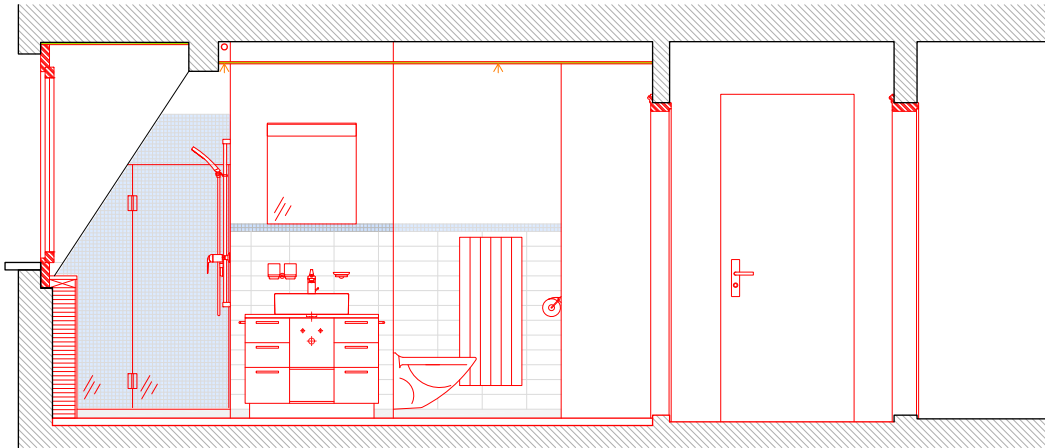
ANSICHT
