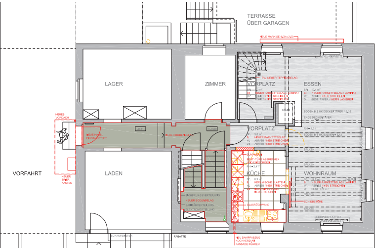
ERDGESCHOSS
