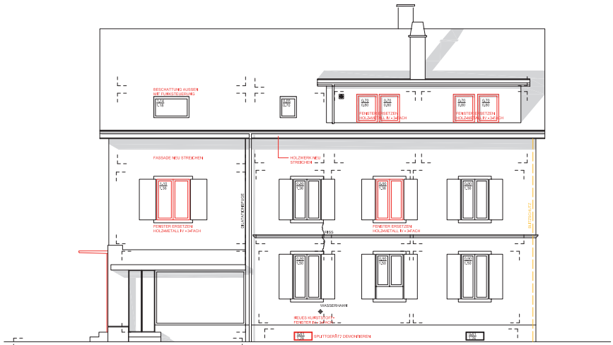
SÜD-WEST-ANSICHT
